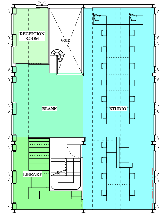
3F PLAN (1/200)
